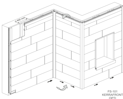
INSTALACE HORIZONTÁLNĚ
