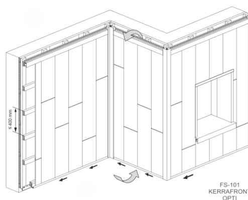
INSTALACE VERTIKÁLNĚ
